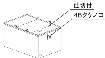
タケノコ溶接組 (1m 3 , 1.5m 3 , 2m 3 )
