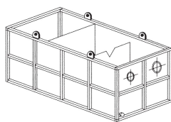
3m 3 , 5m 3 ノッチタンク
