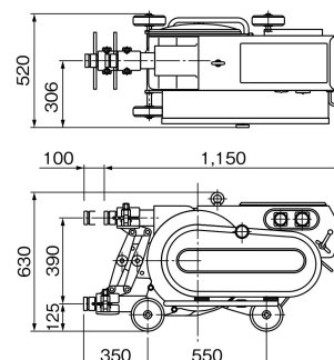
■外形寸法図
